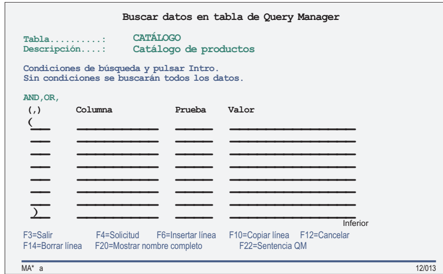
Figura 8. Pantalla de terminal de sistema principal
