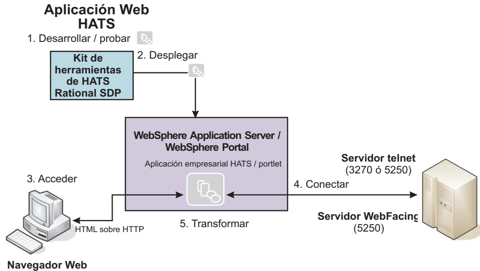
Figura 1. HATS aplicación web
