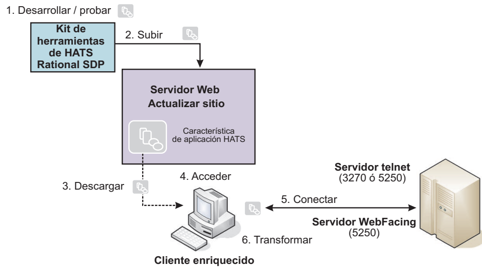
Figura 2. HATS cliente enriquecido aplicación
